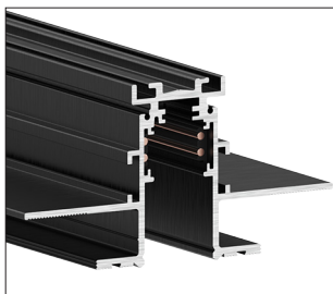
9500-.../B-ST14
