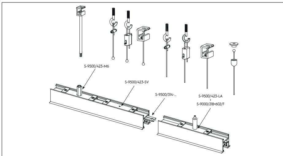
Stoßstellen-Zubehör Accessories for "in row" use junctions
