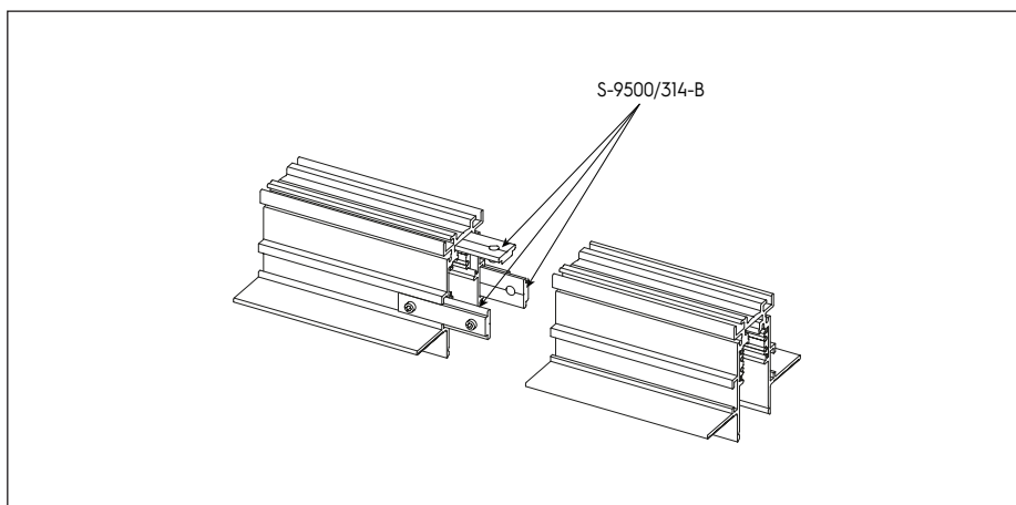
Stoßstellen-Zubehör Accessories for "in row" use junctions
