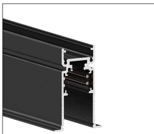
9500-.../B-ST18-E 9500-.../W2-ST18-E
