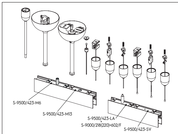
Stoßstellen-Zubehör Accessories for "in row" use junctions
