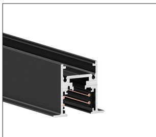
9500-.../B-ST8-E 9500-.../W2-ST8-E
