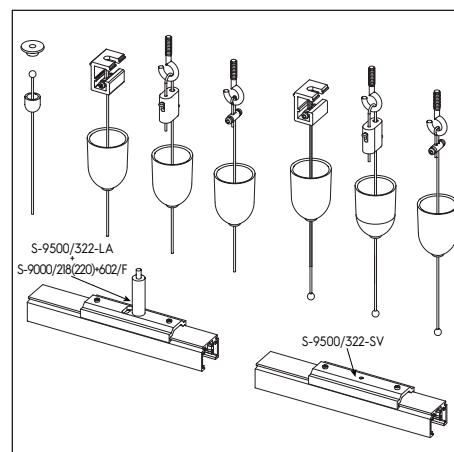
Stoßstellen-Zubehör Accessories for "in row" use junctions
