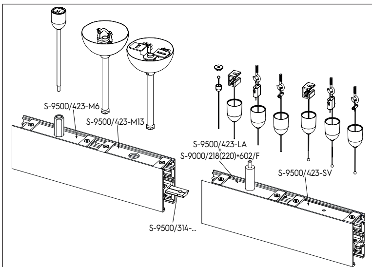
Stoßstellen-Zubehör Accessories for "in row" use junctions
