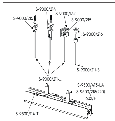
Verstellbares Abhängezubehör (für Stahlseil) Suspension accessories with track adjustment
