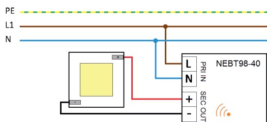
Typisches Schaltbild Typical connection scheme
