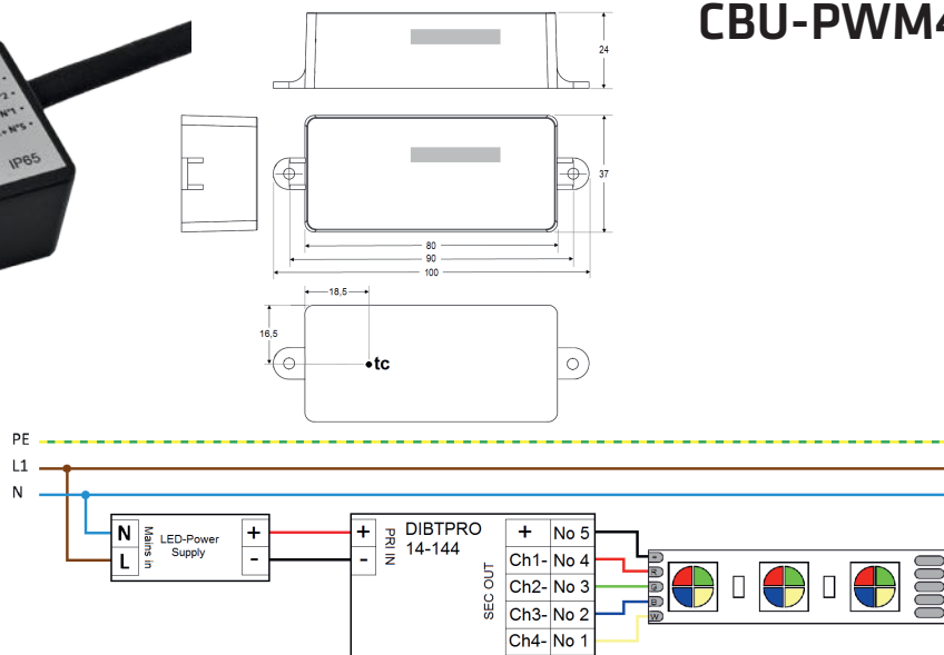
Typisches Schaltbild Typical connection scheme
