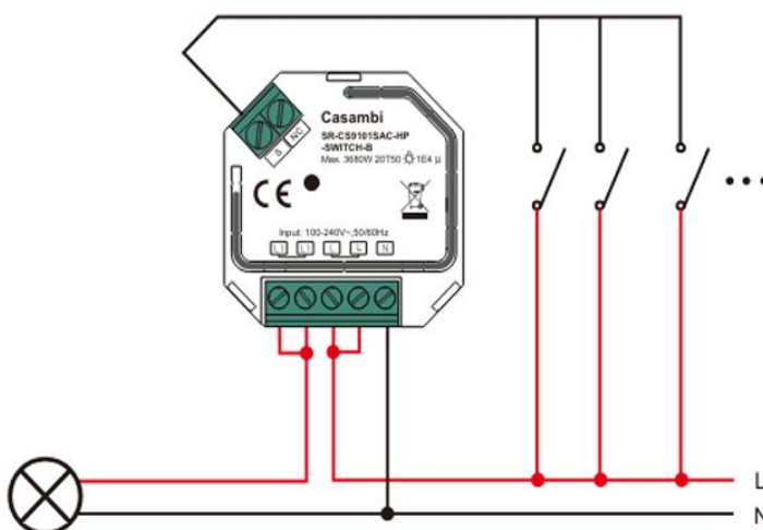
Schaltbild
