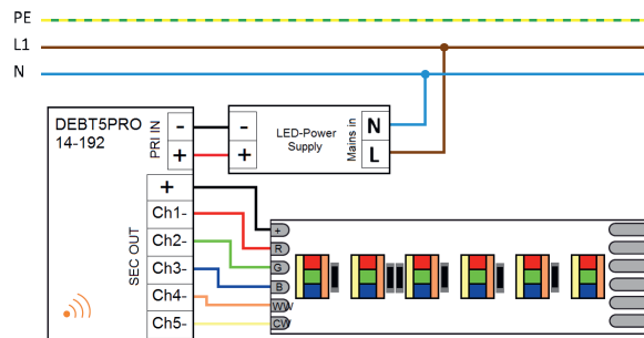
Typisches Schaltbild
