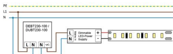
Typisches Schaltbild
