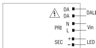
DALI diagram Collegamento DALI
