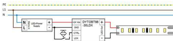
Typisches Schaltbild Typical connection scheme
