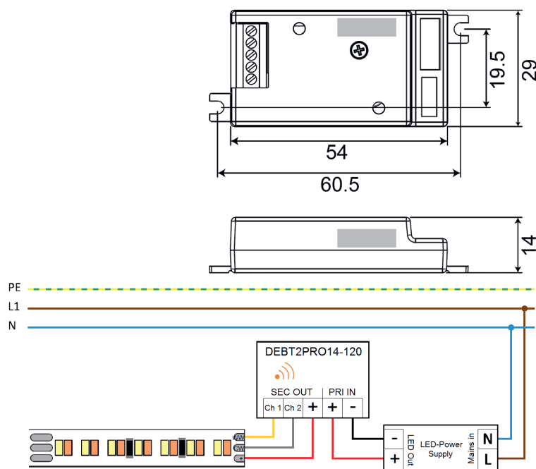
Typisches Schaltbild Typical connection scheme
