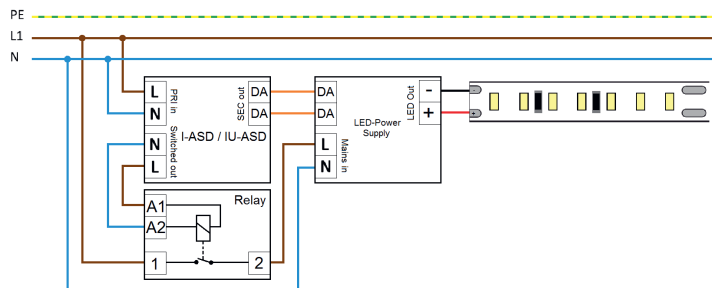
Typisches Schaltbild
