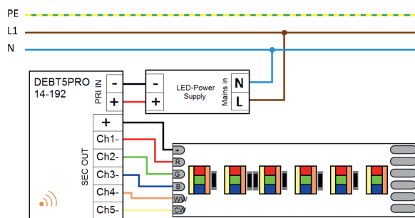
Typisches Schaltbild
