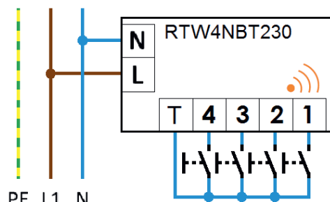
Typisches Schaltbild Typical connection scheme
