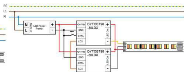
Typisches Schaltbild Typical connection scheme
