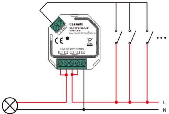
Schaltbild
