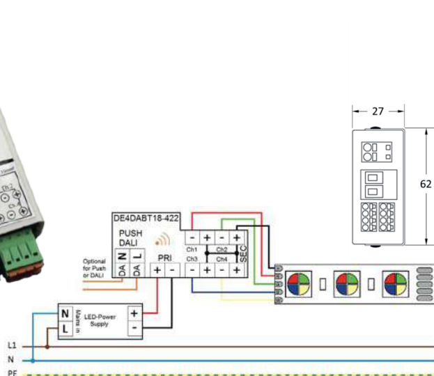
Typisches Schaltbild Typical connection scheme
