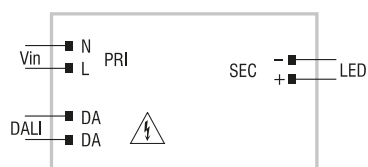
DALI diagram Collegamento DALI
