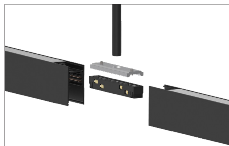
GIUNZIONE IN FILA CONTINUA IN ROW JUNCTION
