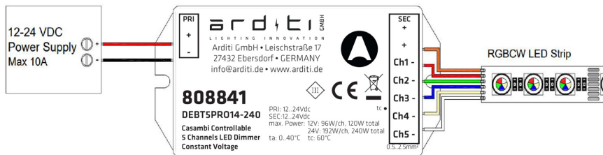
Typisches Schaltbild Typical connection scheme
