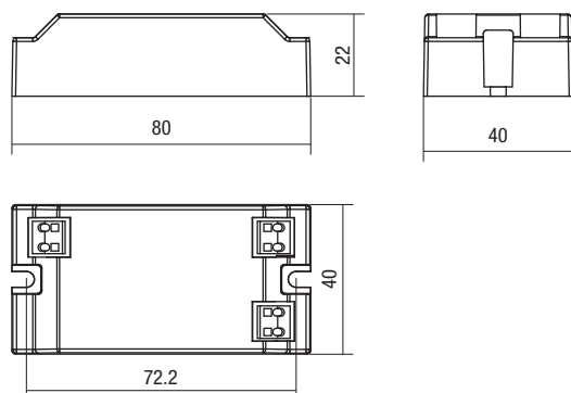
Dimensions (mm) - Maße (mm)
